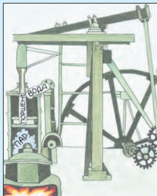
Паровая машина
